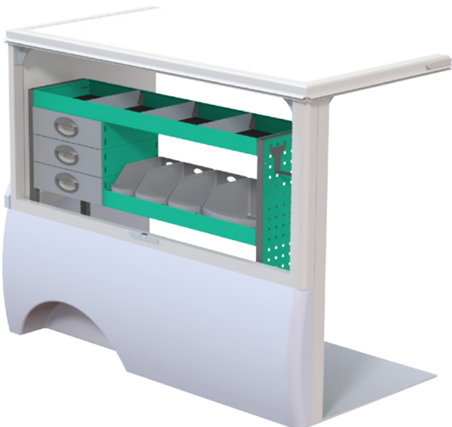
Beställningsnummer F40912 B x D x H 1241 x 300 x 1000 mm • Vikt ca. 30 kg
