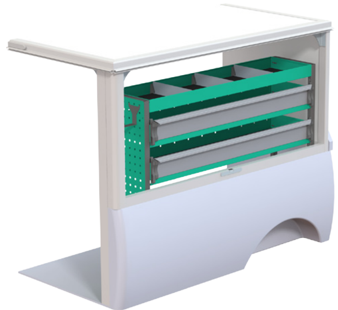
Beställningsnummer F40911 B x D x H 1241 x 300 x 1000 mm • Vikt ca. 28 kg
