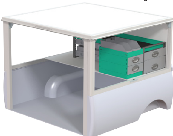
Beställningsnummer F40912 B x D x H 1241 x 300 x 1000 mm • Vikt ca. 30 kg
