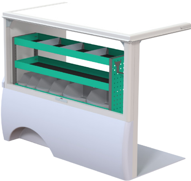
Beställningsnummer F40920 B x D x H 1241 x 300 x 1000 mm • Vikt ca. 26 kg
