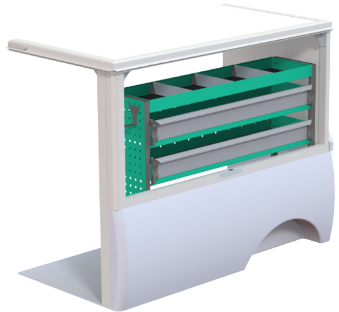
Beställningsnummer F40921 B x D x H 1241 x 300 x 1000 mm • Vikt ca. 28 kg
